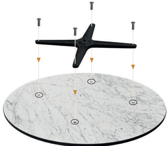
Με ενσωματωμένες υποδοχές στήριξης κεντρικής βάσης τραπέζιου.
